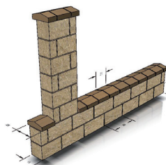
Przęsło ze słupkiem 39 x 19
