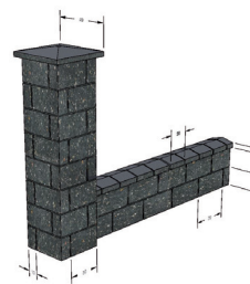
Przęsło ze słupkiem 39 x 39
